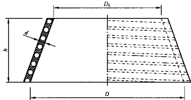
图 6 螺旋缠绕收口锥体结构尺寸示意图
