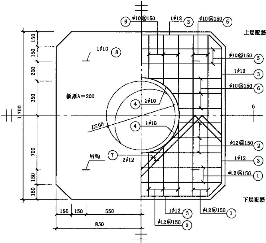
钢筋表
