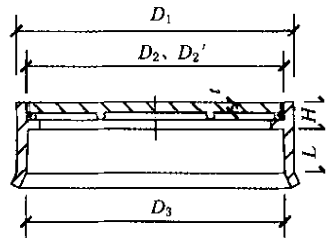
图 A.2 波纹管井筒上配套井盖 表 A.2 双壁波纹管井筒配套井盖尺寸
