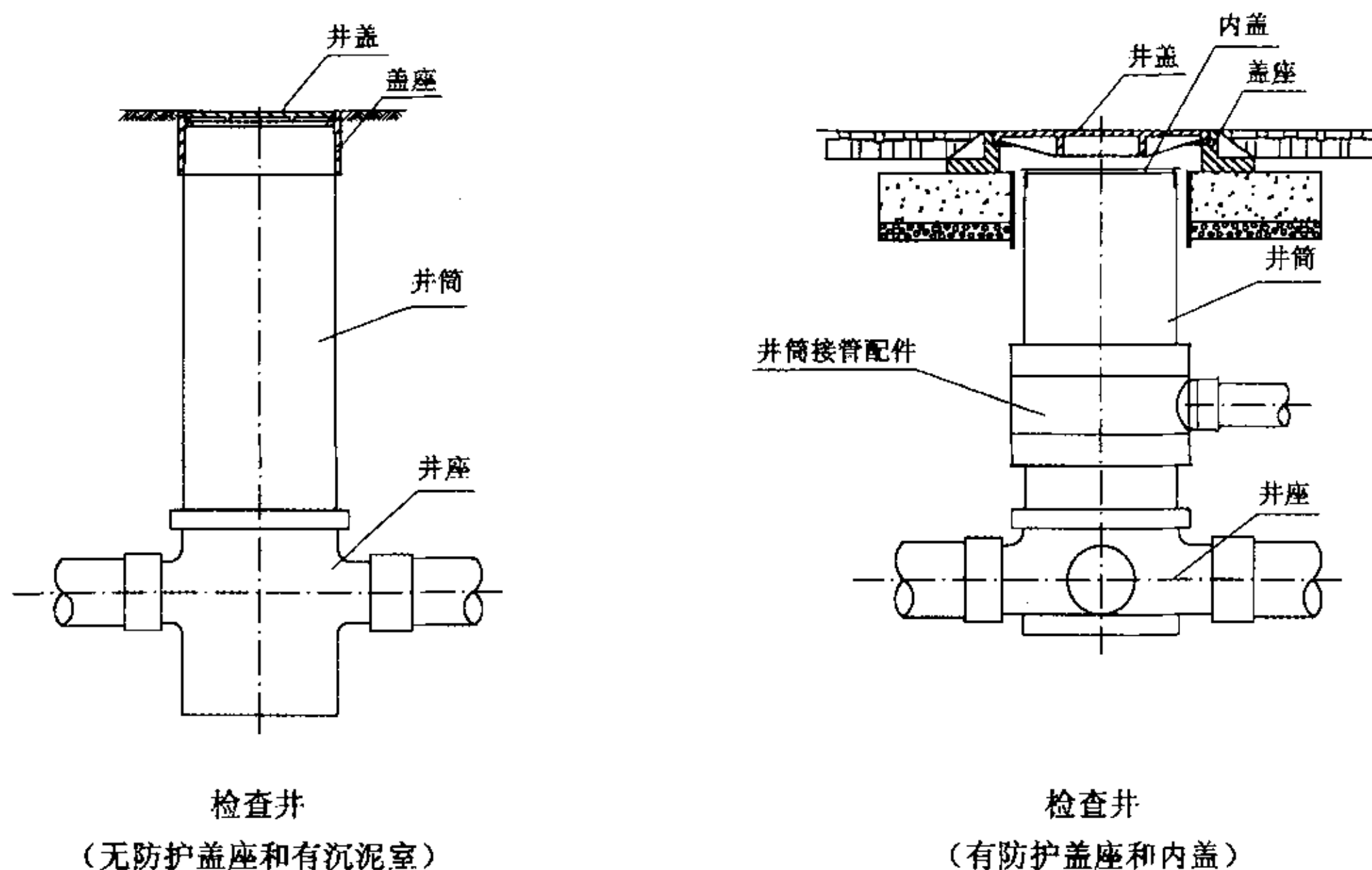
图 1 检查井构成示意图
