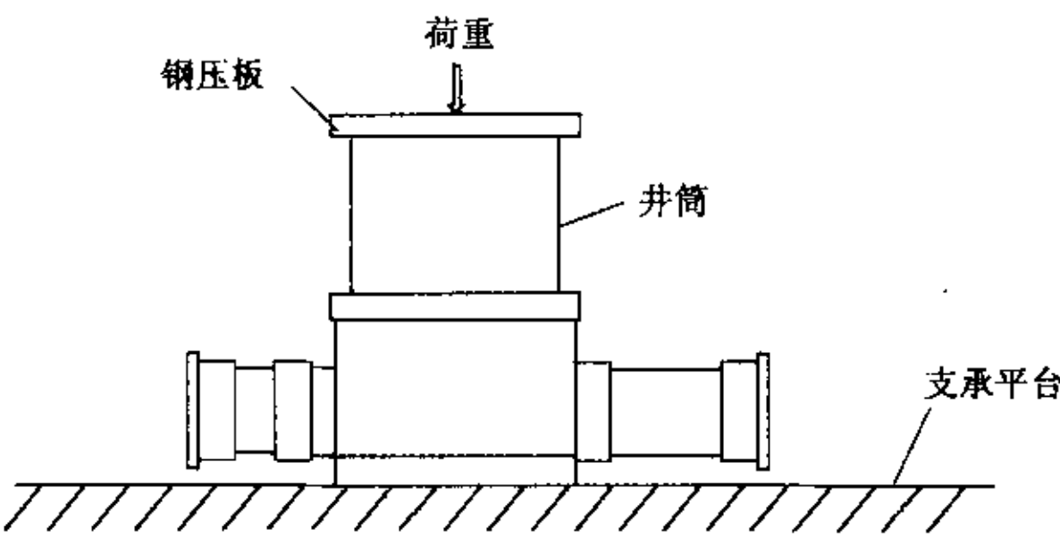
图 7 荷载试验装置
