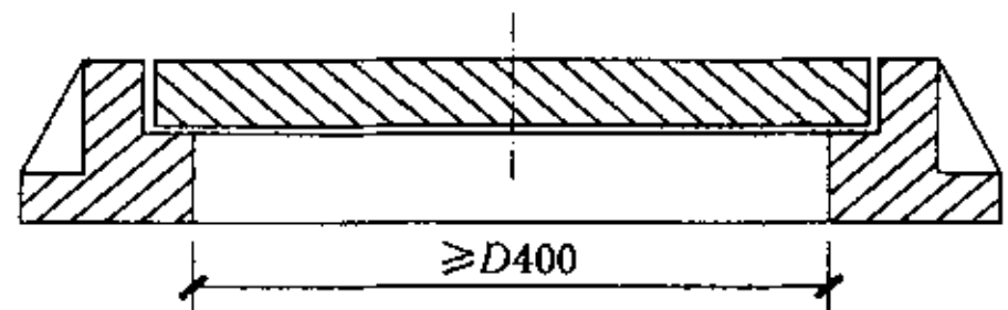
图 A.3 315 防护盖座控制尺寸图
