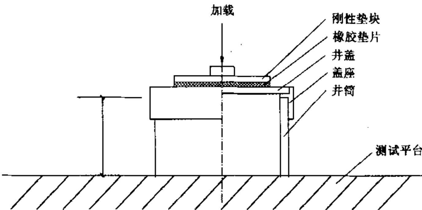
图 A. 7 荷载试验
