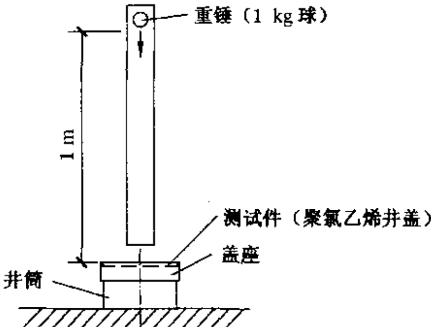
图 A. 8 抗冲击落锤试验
