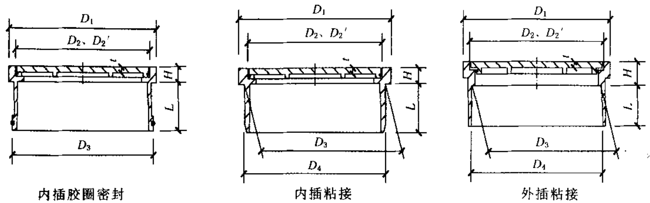
图 A.1 直壁管井筒配套井盖 表 A.1 直壁管井筒配套井盖尺寸
