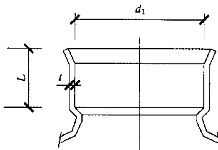
图 4 检查井井座与井筒连接部位不带窝槽弹性密封承口示意图
