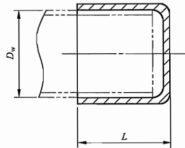
图 9 管帽钎焊管件
