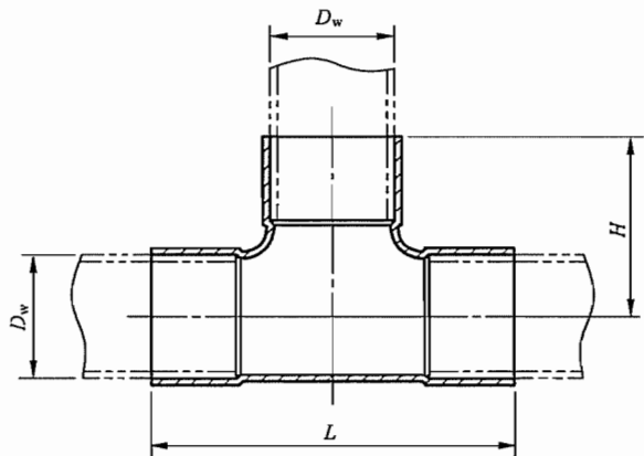
图 2 等径三通钎焊管件
