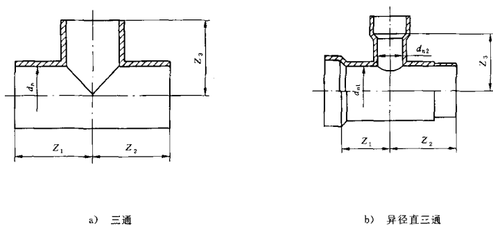
图 B.2 典型三通示意图
