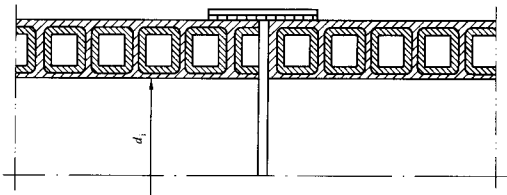
图 C.6 热收缩套连接示意图
