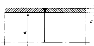
图 C.5 V型焊接连接示意图
