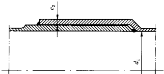
图 C.3 承插口焊接连接示意图
